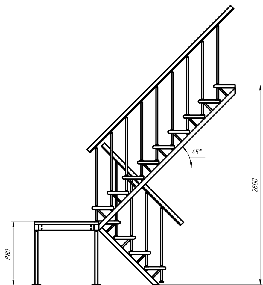
Рисунок 2. Лестница внутриквартирная правозаходная ЛЕС-06П.
