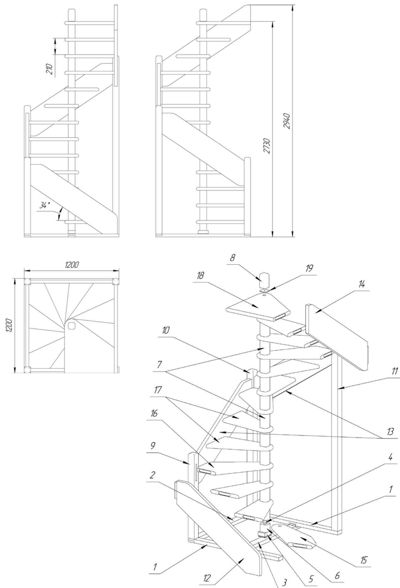
Рисунок 1. Лестница внутриквартирная ЛЕС-216.
